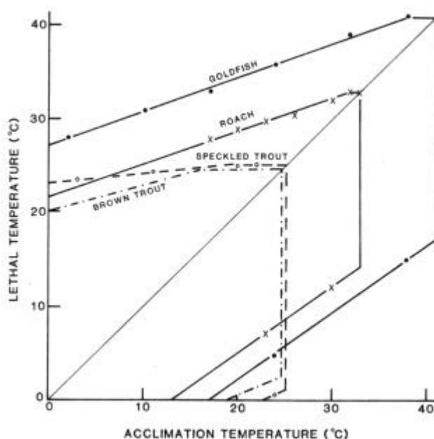
Abb. 2: Toleranzdiagramm für Goldfisch (goldfish), Rotaugen (roach), Bachsaibling (speckled trout) und Forelle (brown trout) (aus Elliott 1981).
