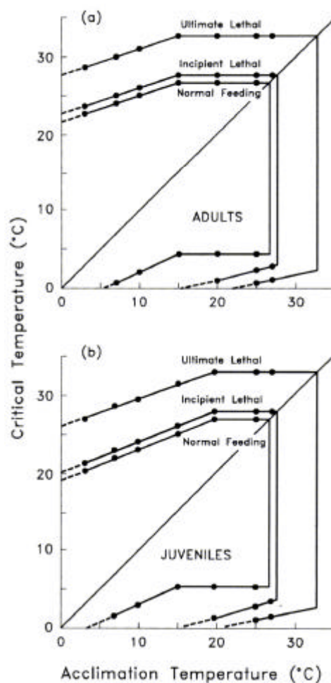
Abb. 10: Polygon der Temperaturtoleranz für adulte (a) und juvenile (b) Gropfen (aus Elliott 1995)
